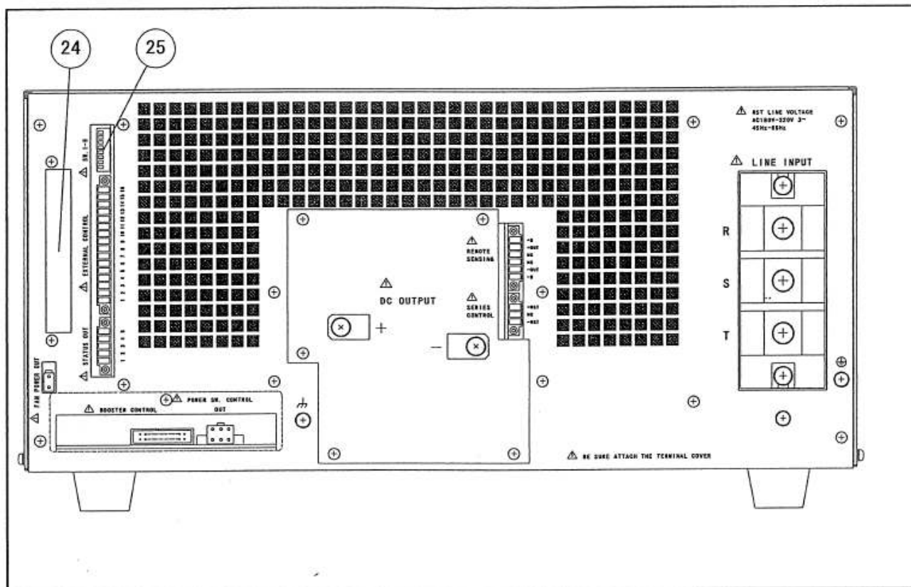
図1-2 リアパネル
