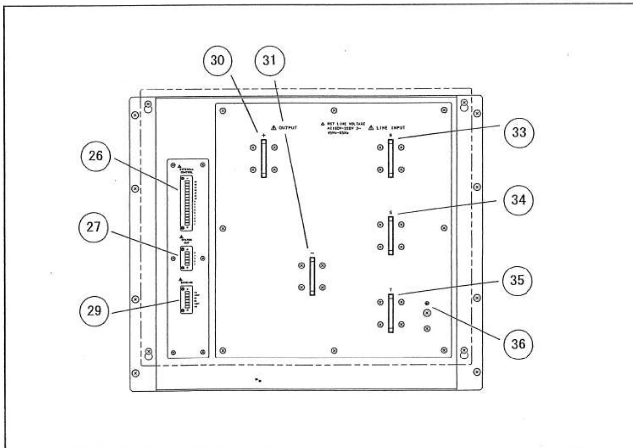
図1-3 架背面・端子図
