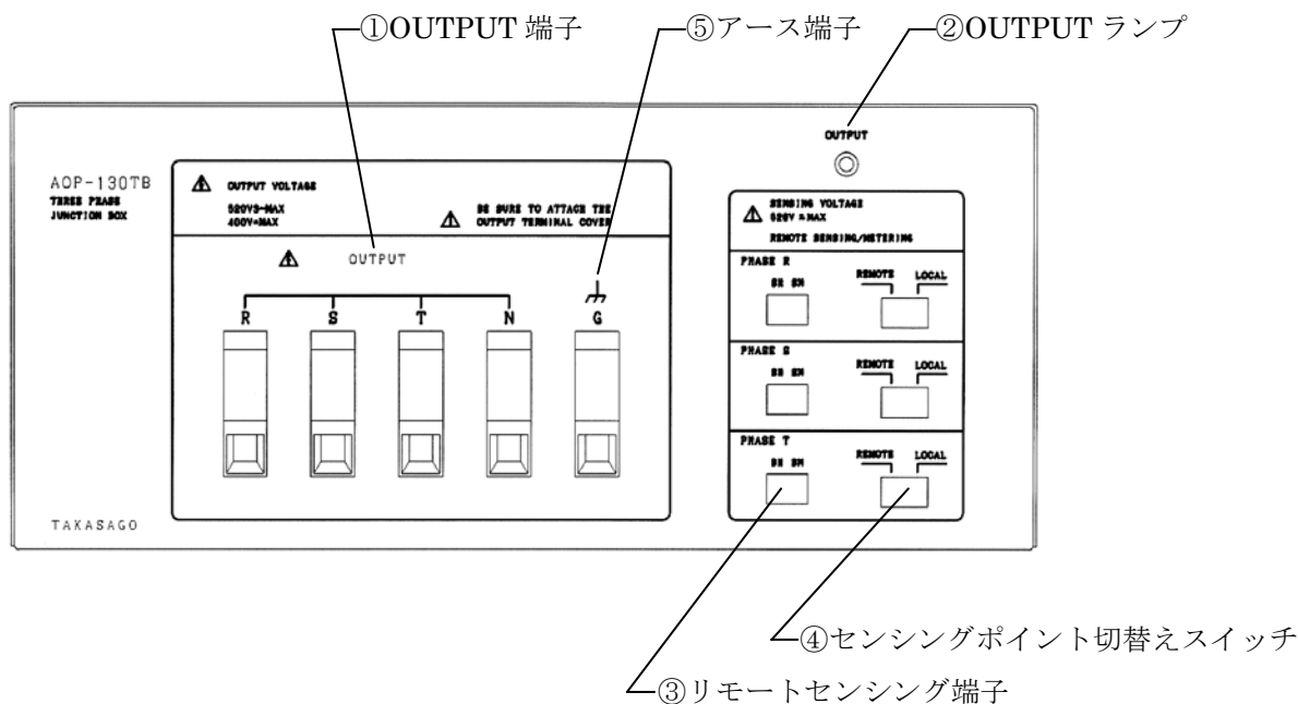
図5. 出力部 AOP-130TB詳細図
