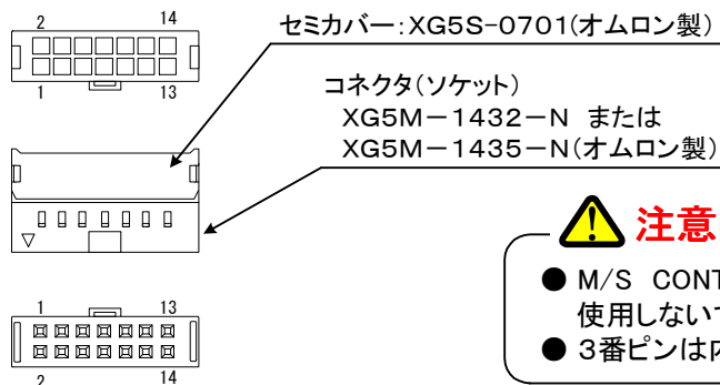
外部接点による、出力のON/OFF
