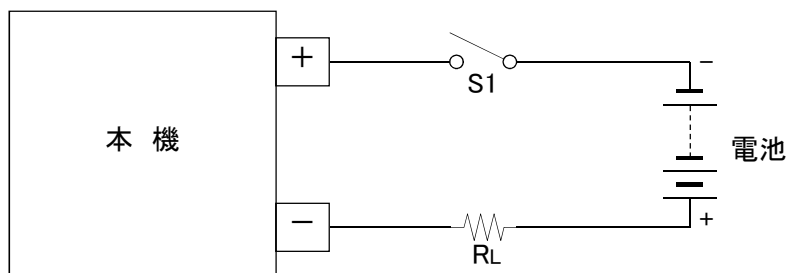
電池の定電流放電
