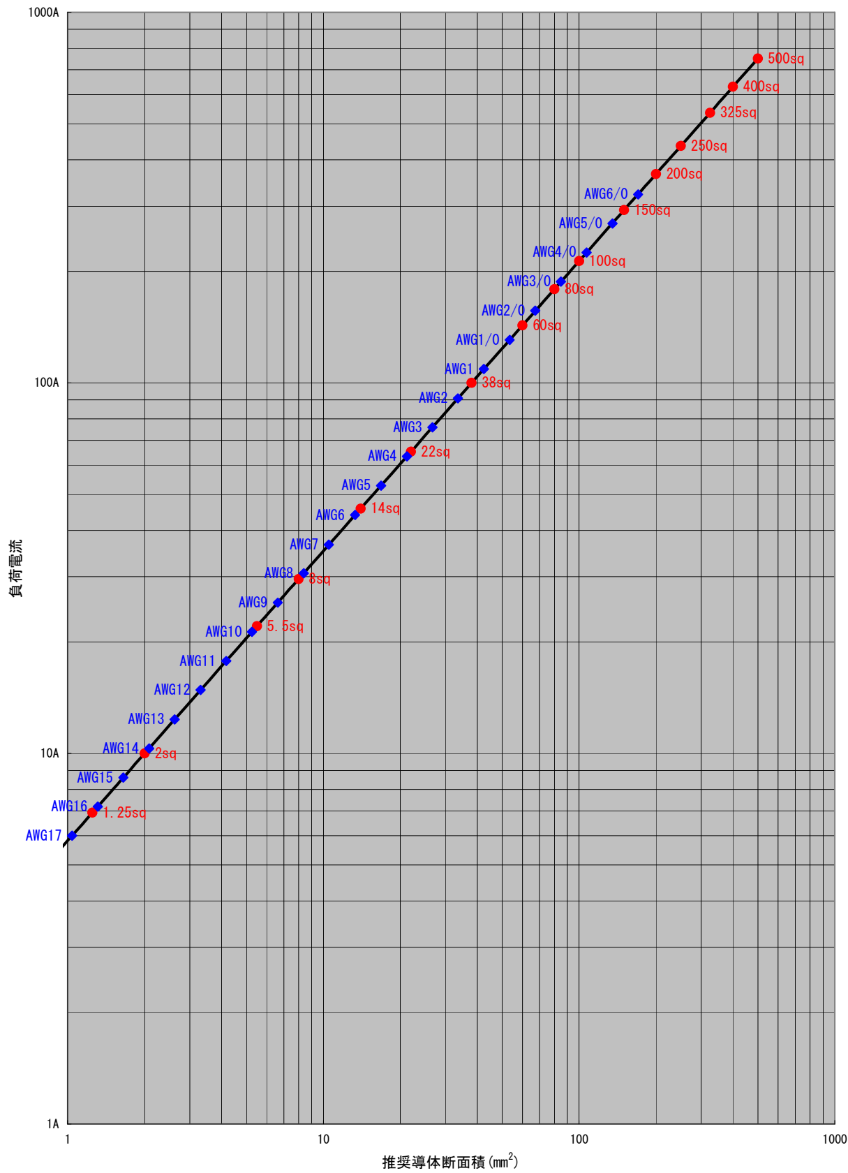
付録 負荷電流 対 推奨導体面積
