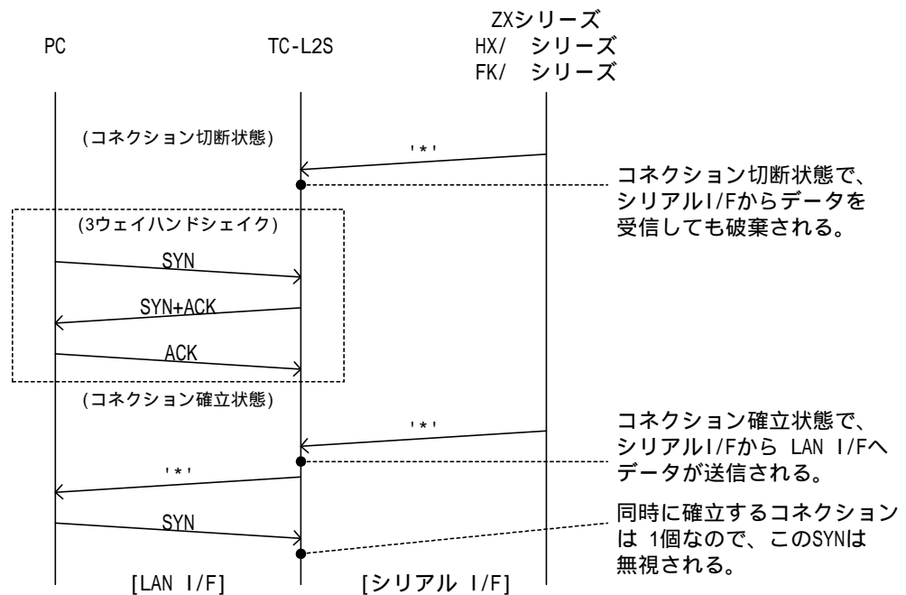
(図 . TC-L2S の接続)
