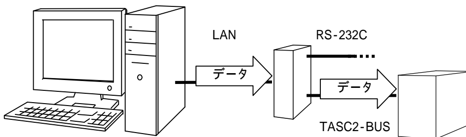
(図.LAN TASC2-BUS) RS-232C の接続未検出なので、TASC2-BUS にデータ送信する。
