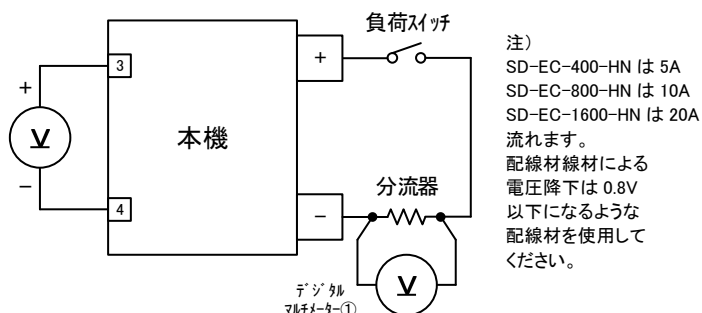
構成回路
