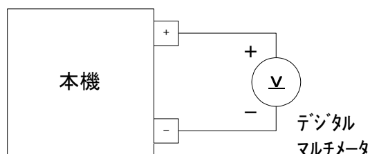
校正回路
