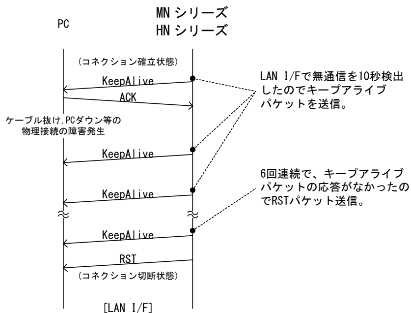
(図. キープアライブパケットによる物理接続監視)
