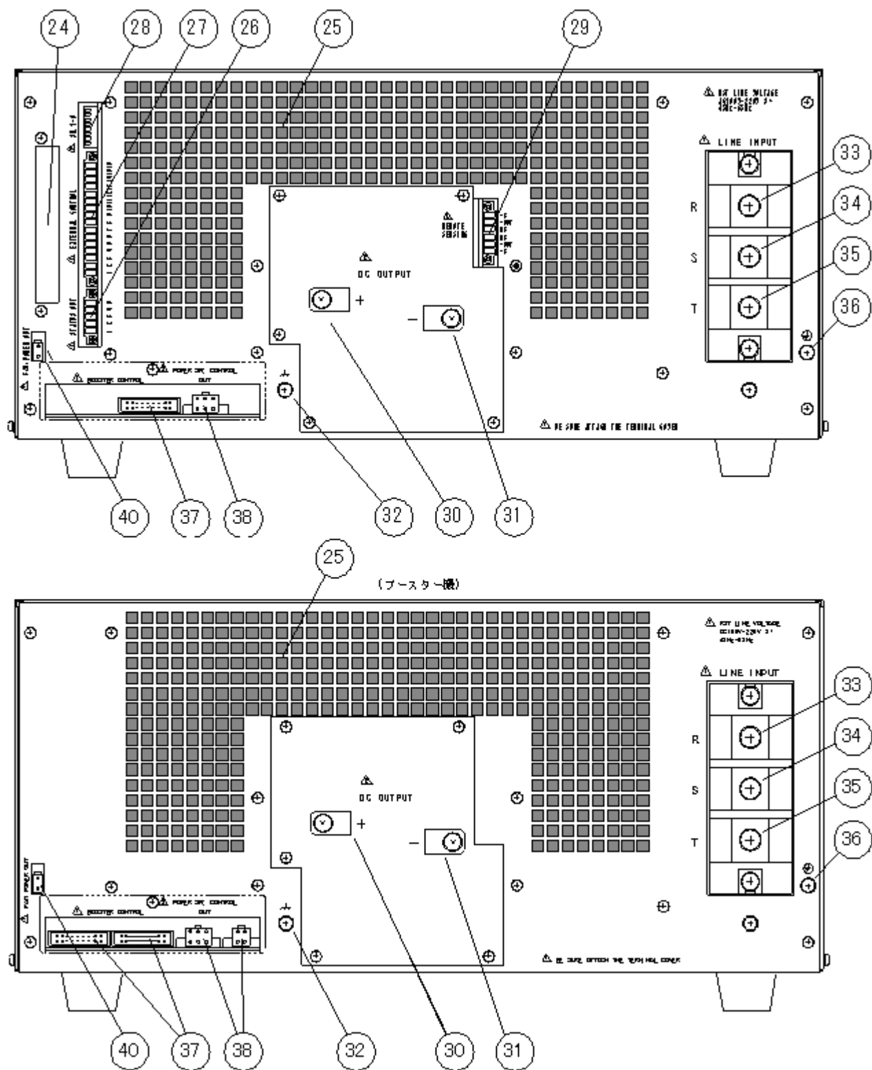
図1-2 リアパネル
