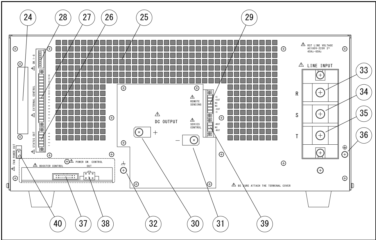
図1-2 リアパネル
