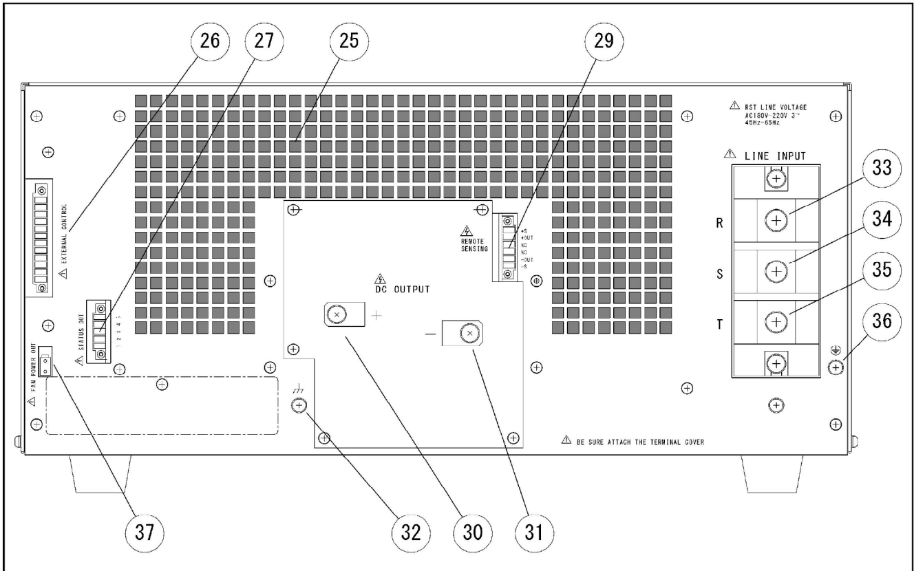
図1-2 リアパネル
