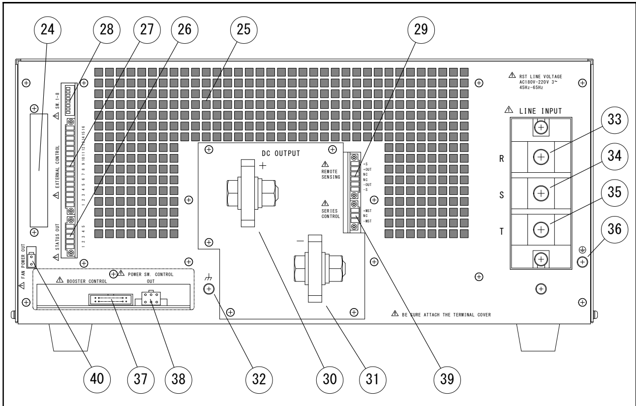
図 1-2 リアパネル
