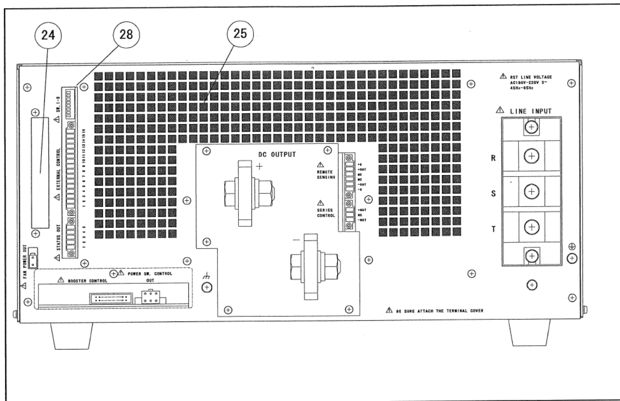
図1-2 リアパネル
