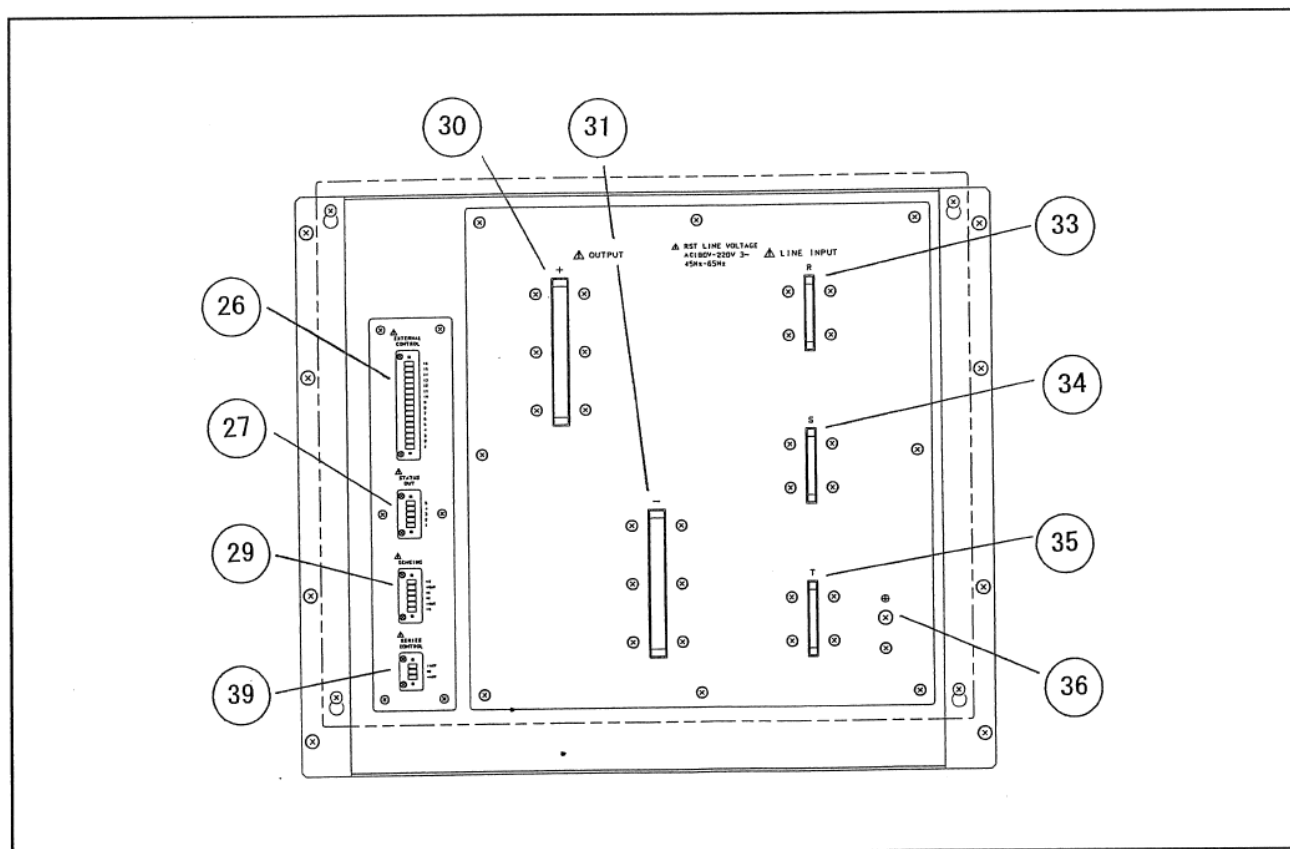
図1-3 架・入出力端子
