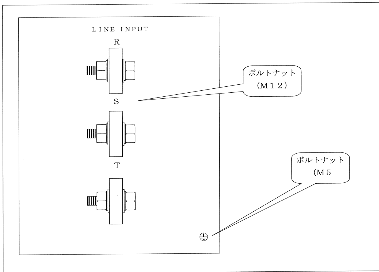
図2-1 動作電源の接続
