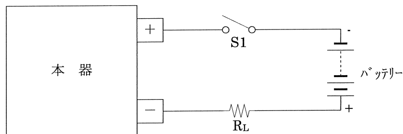
図5-3 バッテリー放電の接続
