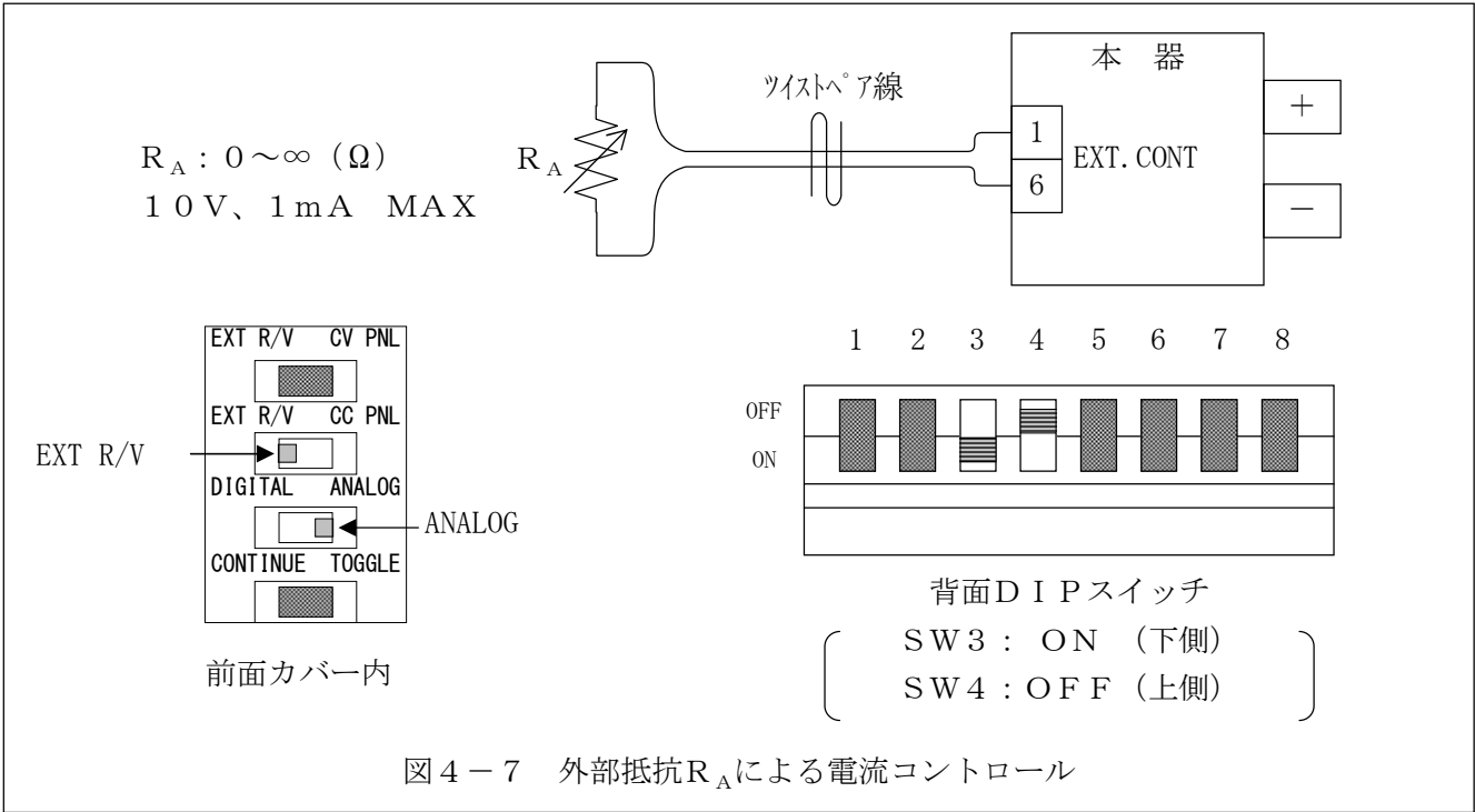
図 4－7 のように配線し、背面DIPスイッチと前面カバー内のスイッチを設定してください。
