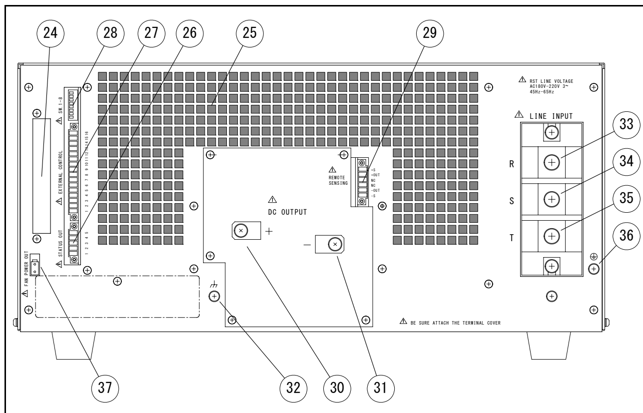
図1-2 リアパネル
