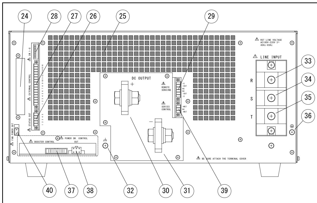
図1-2 リアパネル
