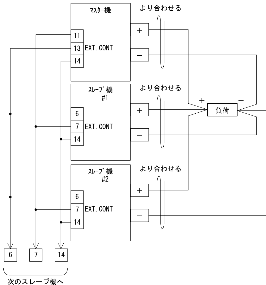
図4-17 マスタースレーブ並列運転
