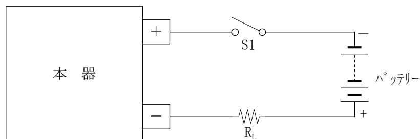
図5-3 バッテリー放電の接続
