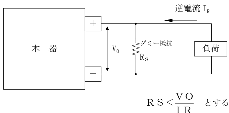
図5－4 ダミー抵抗による逆電流の吸収
