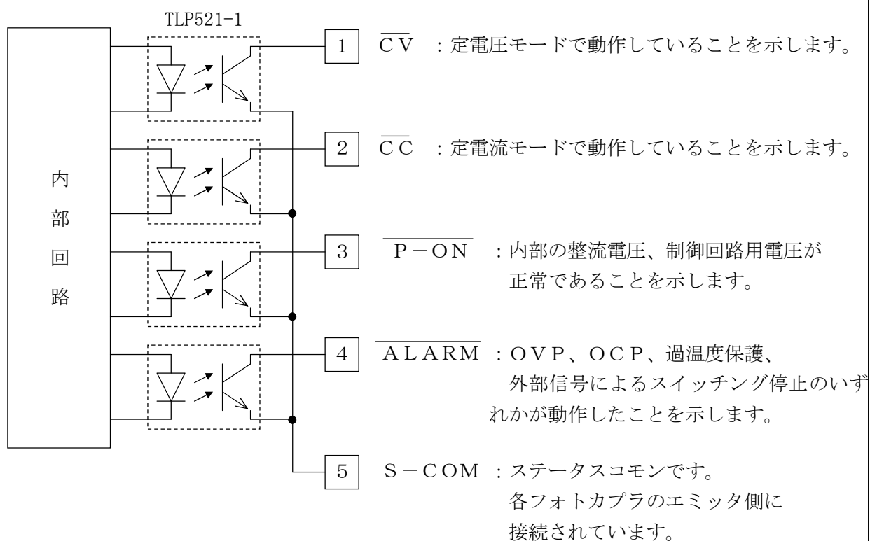
図4-13 ステータス出力回路
