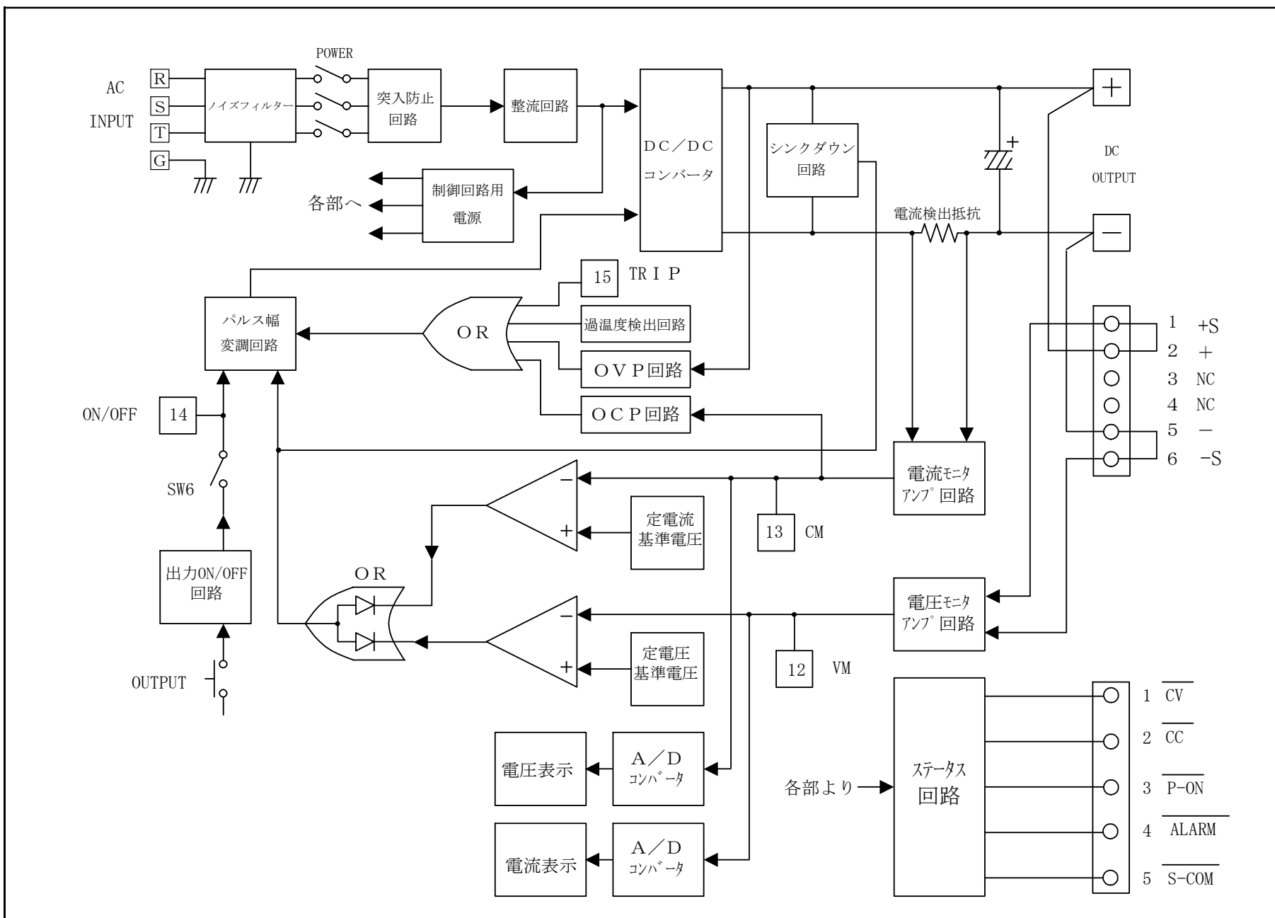
付録2 回路ブロック図
