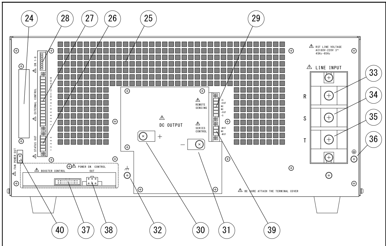
図1-2 リアパネル (マスターユニット)
