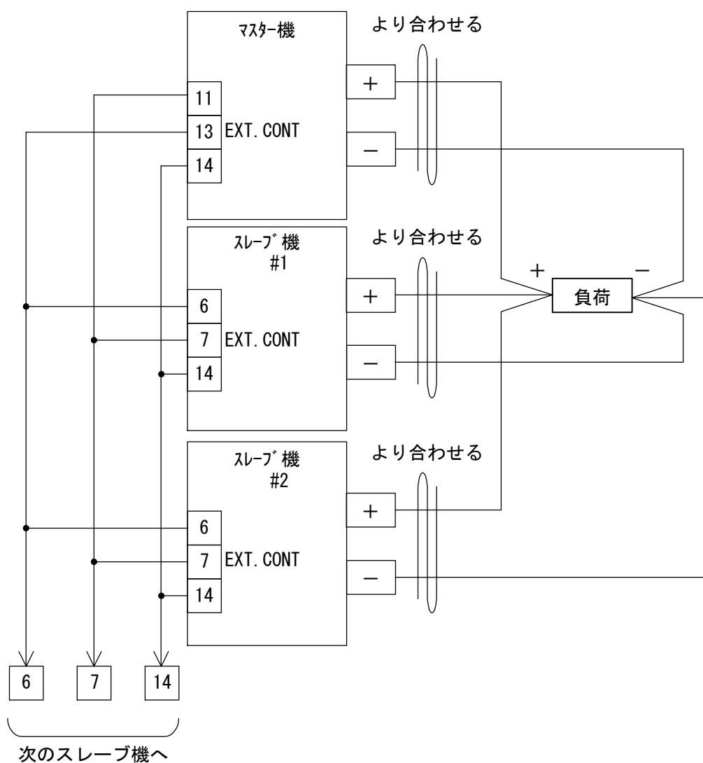
図4-17 マスタースレーブ並列運転
