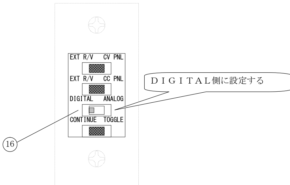
図6-2 デジタルコントロールの設定
