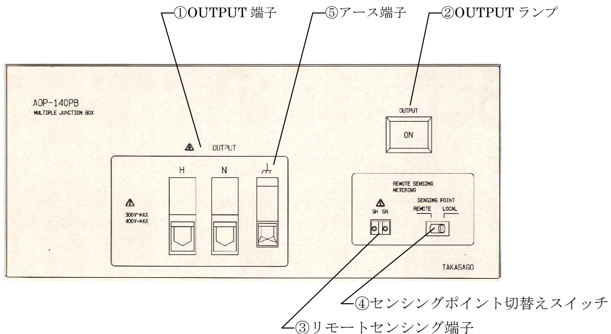
図5. 出力部 AOP-140PB詳細図
