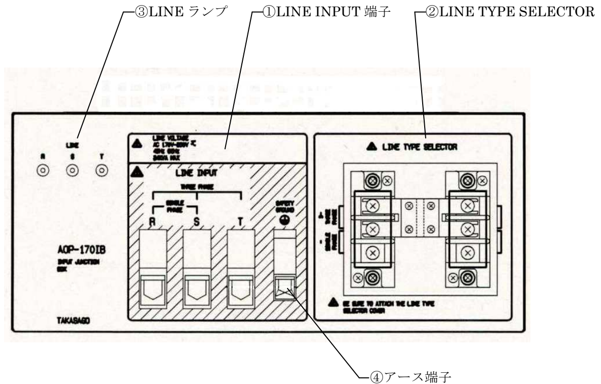
図6. 入力部 AOP-170IB詳細図
