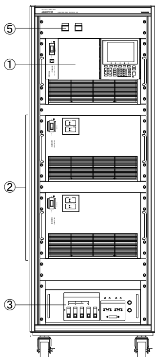
図1. 前面側
