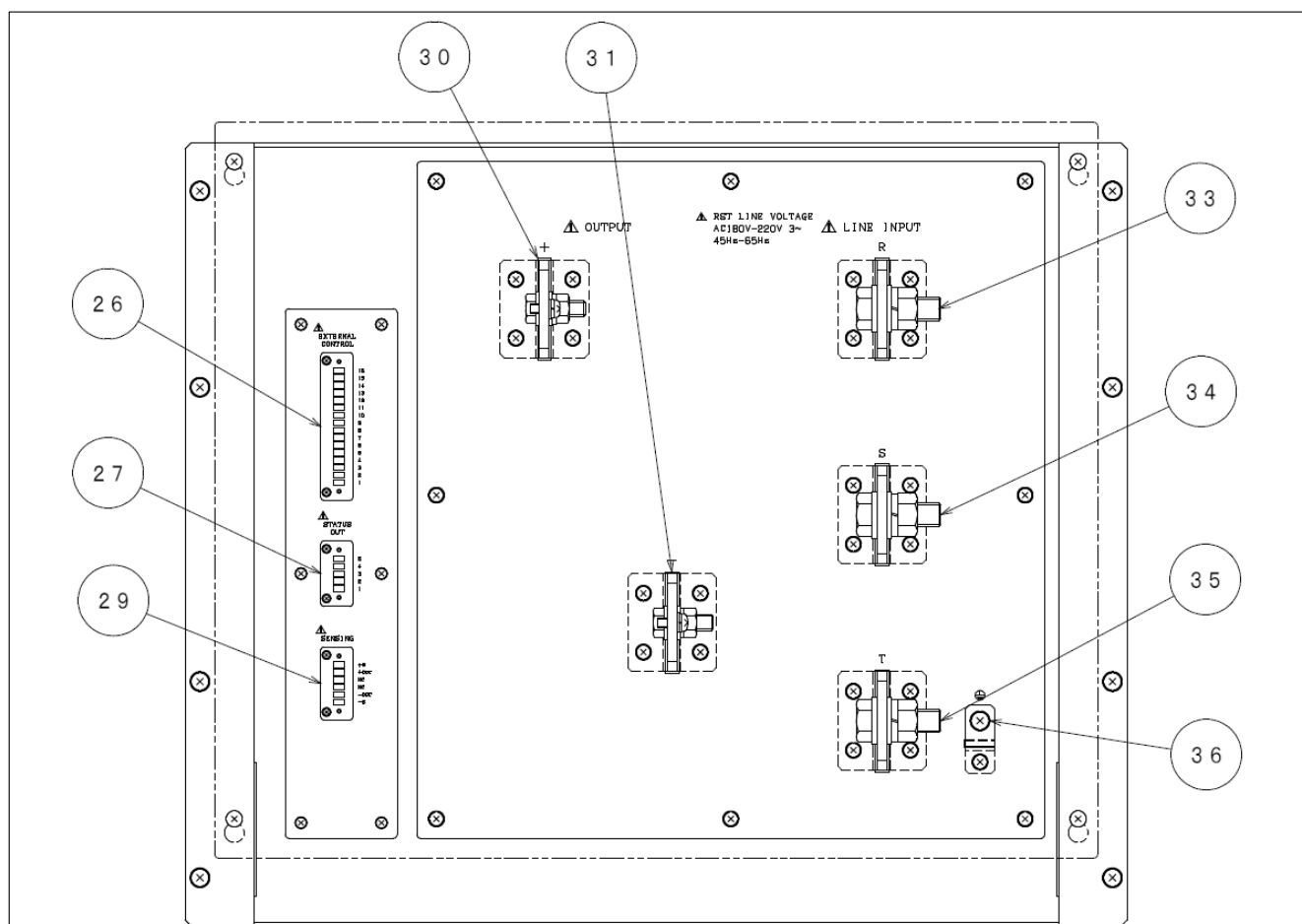
図1-3 架背面 端子図
