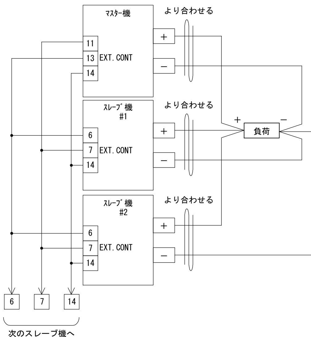
図4-14 マスタースレーブ並列運転
