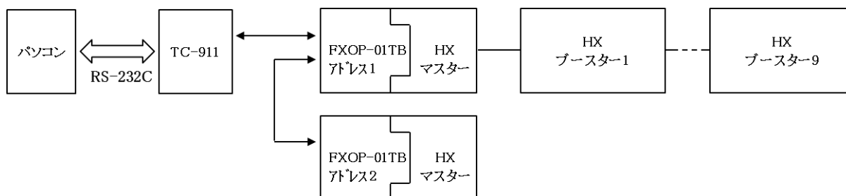
図 4-8 並列接続例
