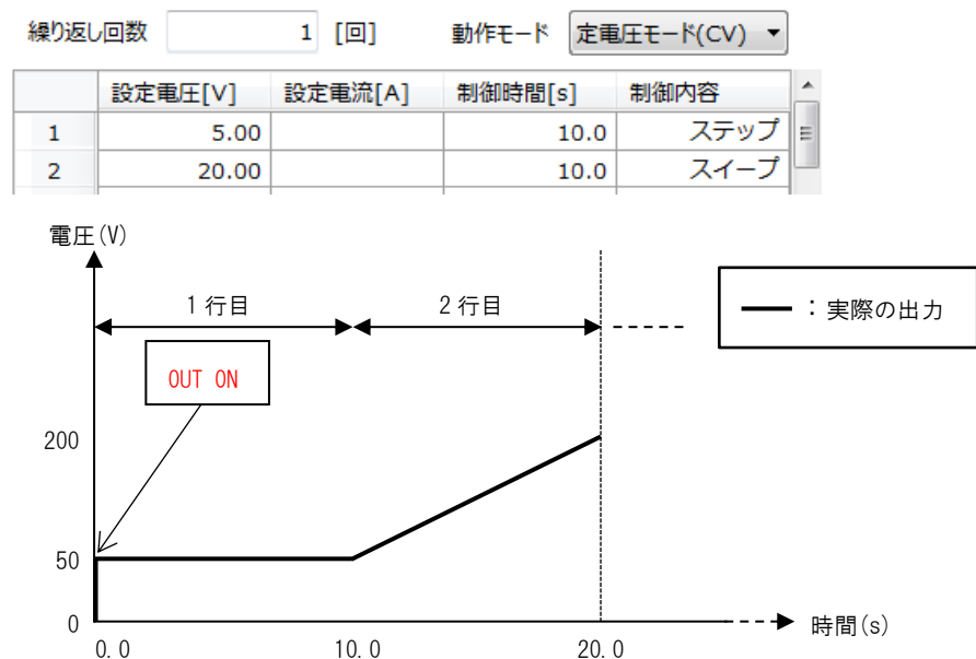
図 7-10 スweep動作例(定電圧モード(CV)設定時)
