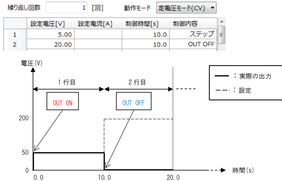
図 7-11 OUT OFF 動作例(定電圧モード(CV)設定時)
