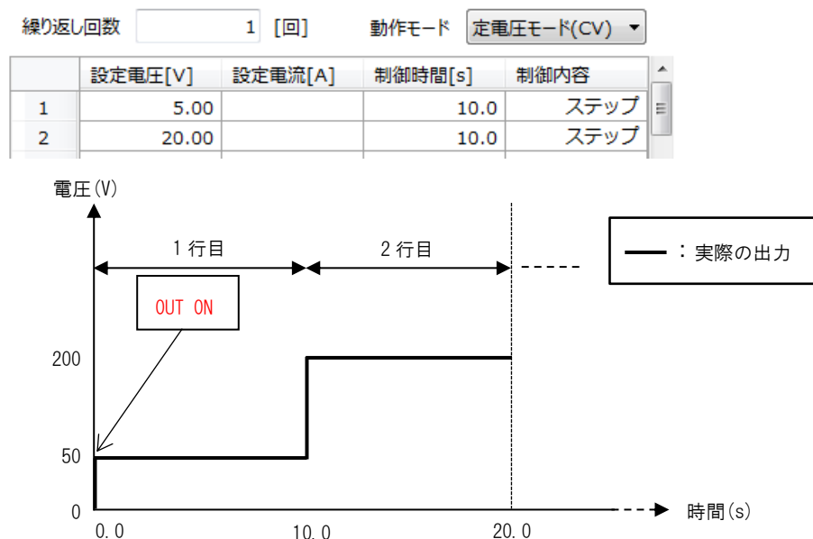
図 7-9 ステップ動作例(定電圧モード(CV)設定時)
