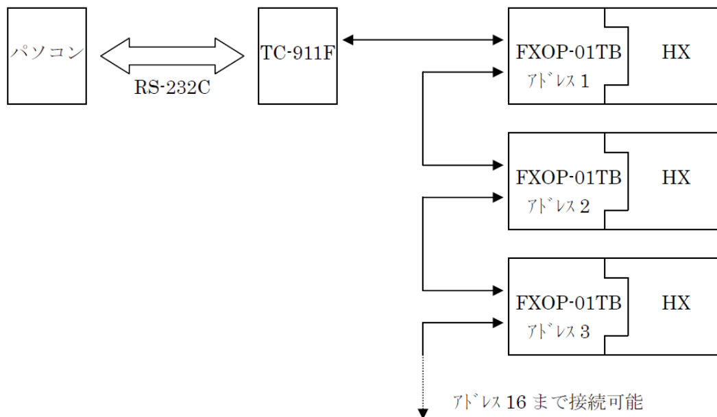
図 5-1 マルチ接続図
