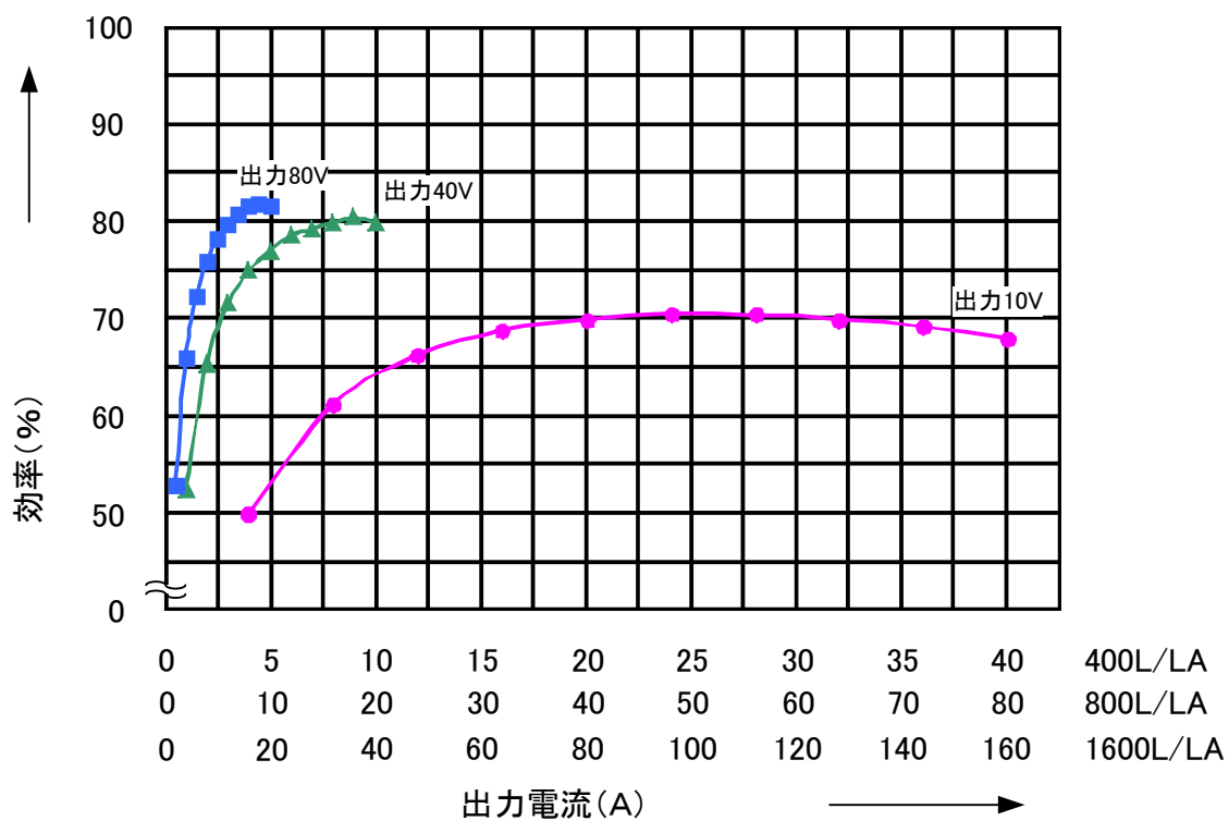
付録② 出力電流 対 効率
