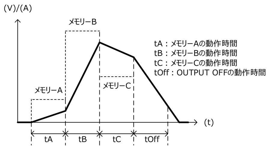
(例 2)スルーレートで目標設定値に到達しない場合の動作
