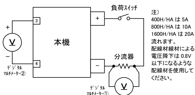
構成回路
