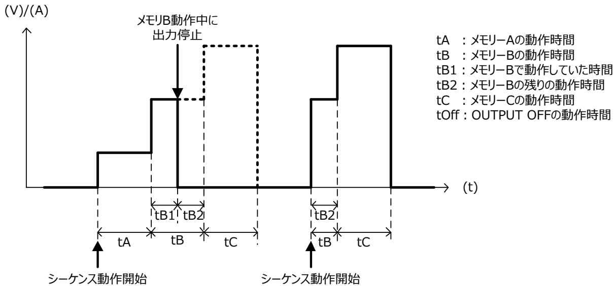
図 3-7 コンティニューモード有効時のシーケンス動作
