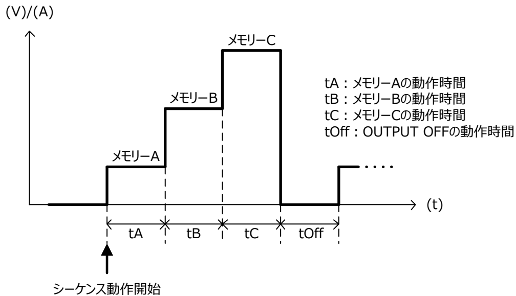
図3-6 シーケンス動作時の出力波形
