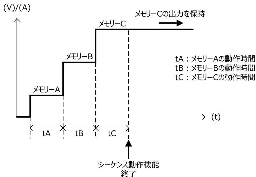
図 3-8 シーケンス有限回数終了後の OUTPUT OFF 無効時（設定項目 24 = 0）
