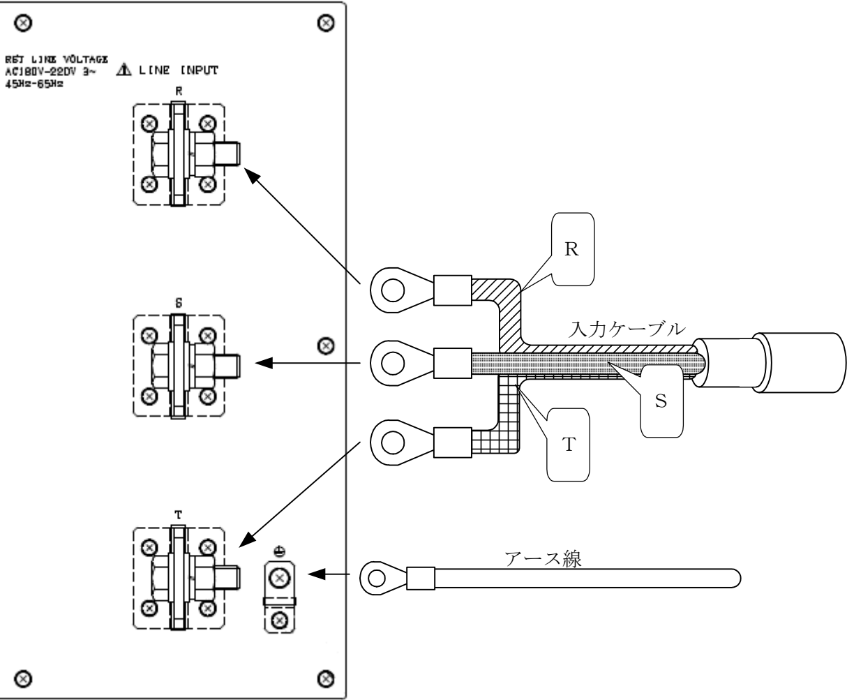
図2-1 動作電源の接続
