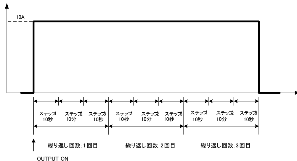
電流波形
