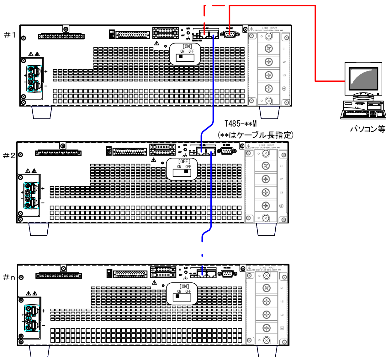
複数の HX-S-G2 シリーズをパソコンで制御する
