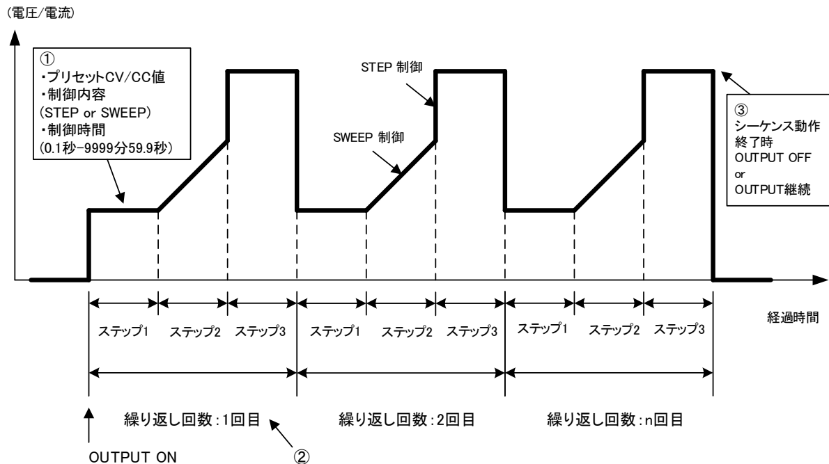
シーケンス動作機能概念図
