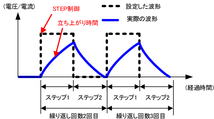
プログラミング時間 > 制御時間の際の波形イメージ図
