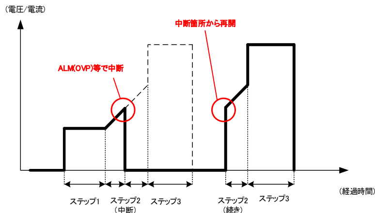
シーケンス動作継続イメージ図
