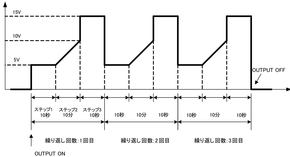
電圧波形
