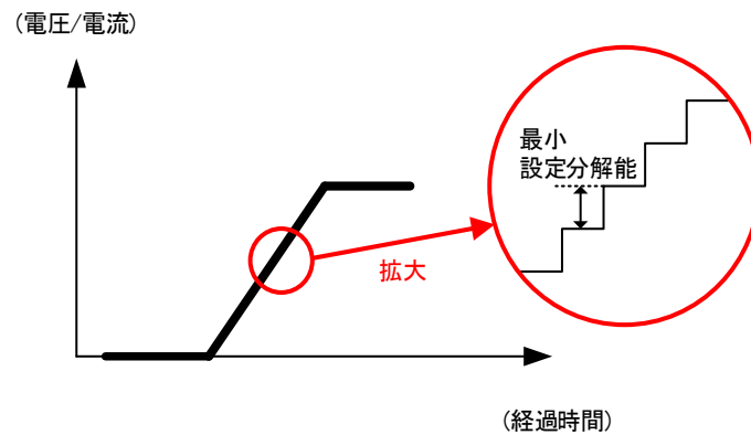
SWEEP 制御イメージ図
