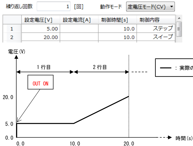
図 7-10 スweep動作例 (定電圧モード (CV) 設定時)
