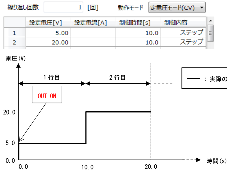
図 7-9 ステップ動作例 (定電圧モード (CV) 設定時)
