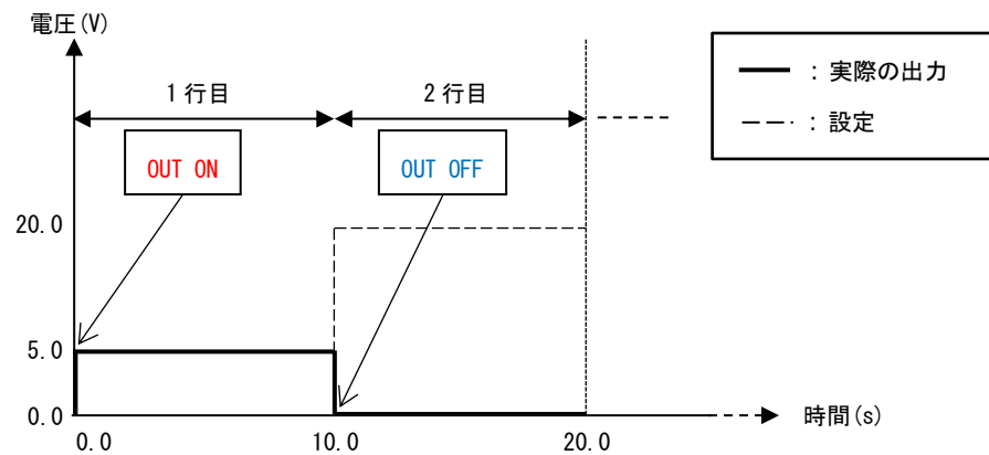
図 7-11 OUT OFF 動作例 (定電圧モード (CV) 設定時)
