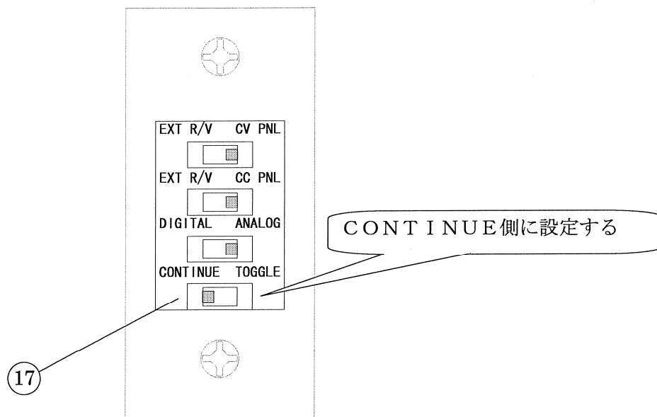
図3-2 『CONTINUE-TOGGLE』の設定
