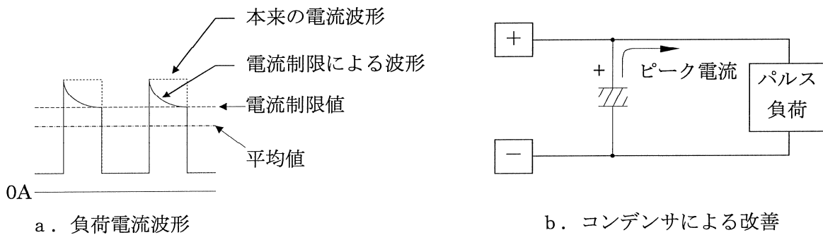
図5-6 パルス逆電流の場合
