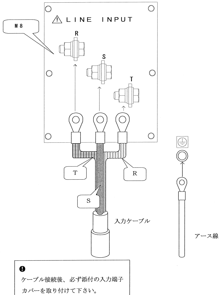
図2-1 動作電源の接続
