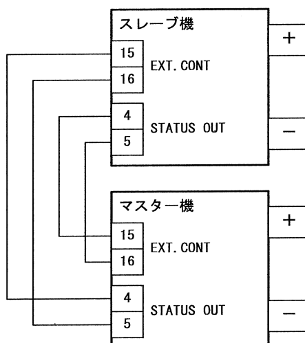
図 4-15 アラーム信号による相互スイッチング停止
