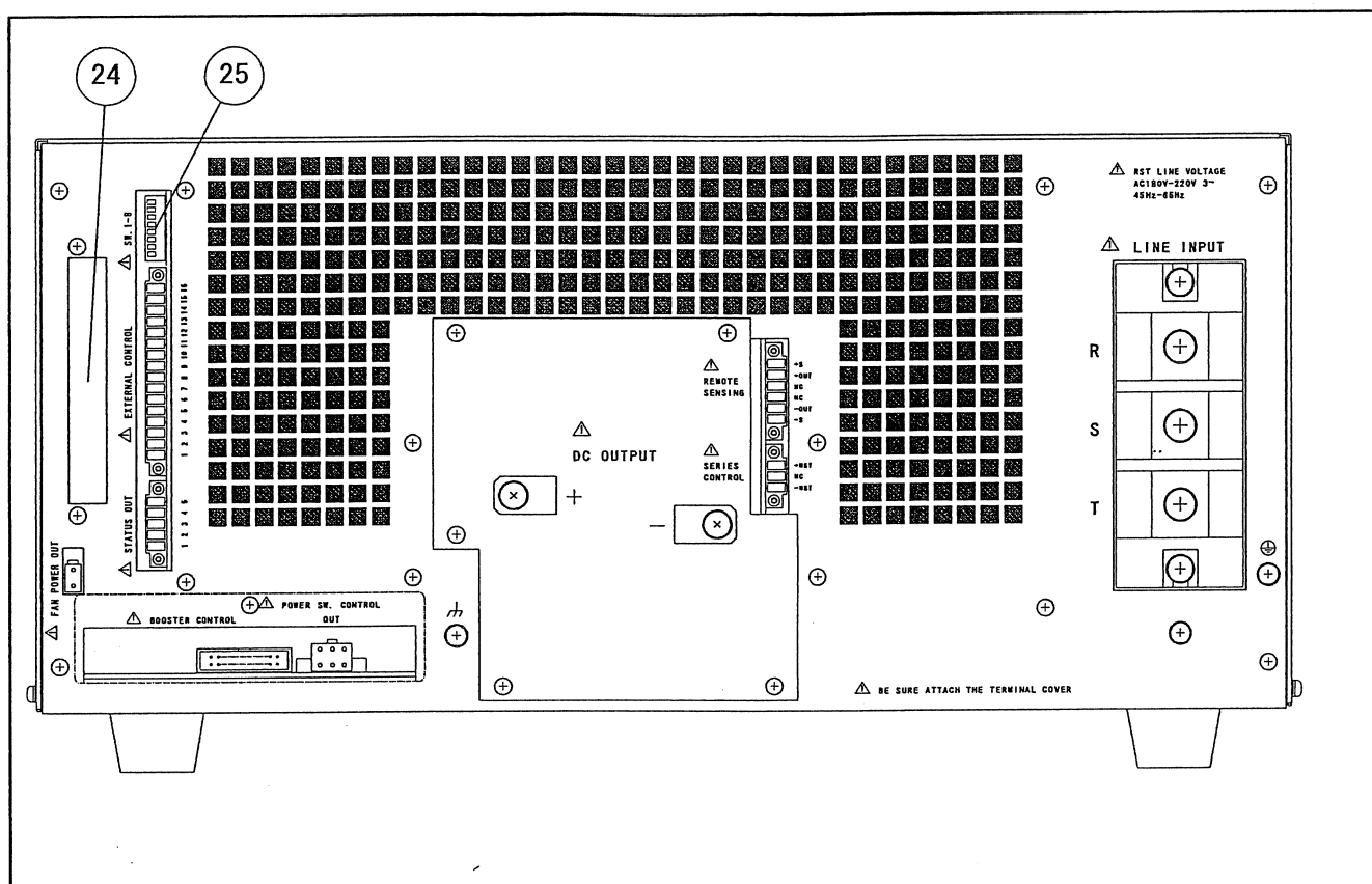
図 1-2 リアパネル
