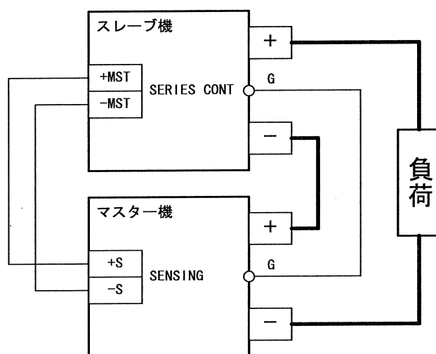
図 4-14 マスタースレーブ並列運転
