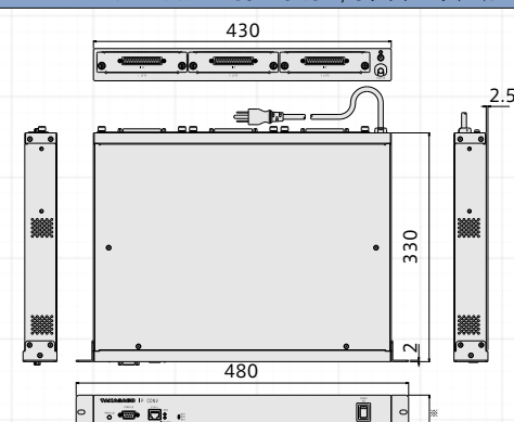
IP Converter (IP-S/3・IP-SE/3) / IP Converter I/Oテレメータ (IP-T/3・IP-TE/3)
