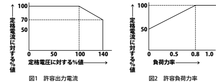
図1 許容出力電流
