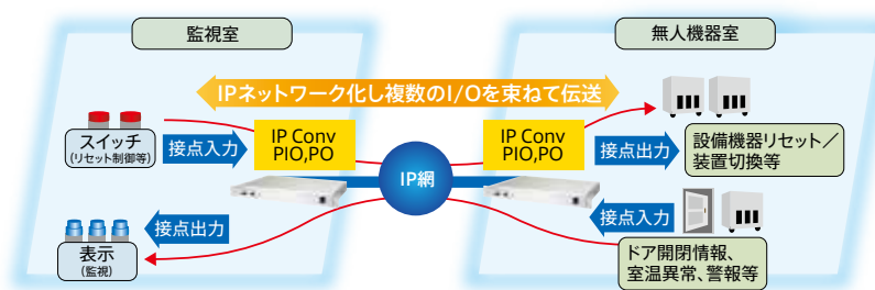
IP Converter I/O伝送システム構成
