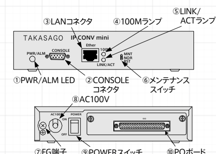
PIOボード (IP-I/PIO/16/8)
