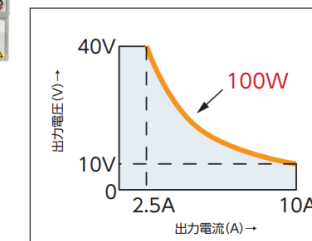
【出力電圧・電流範囲】 KX-S-100-L
